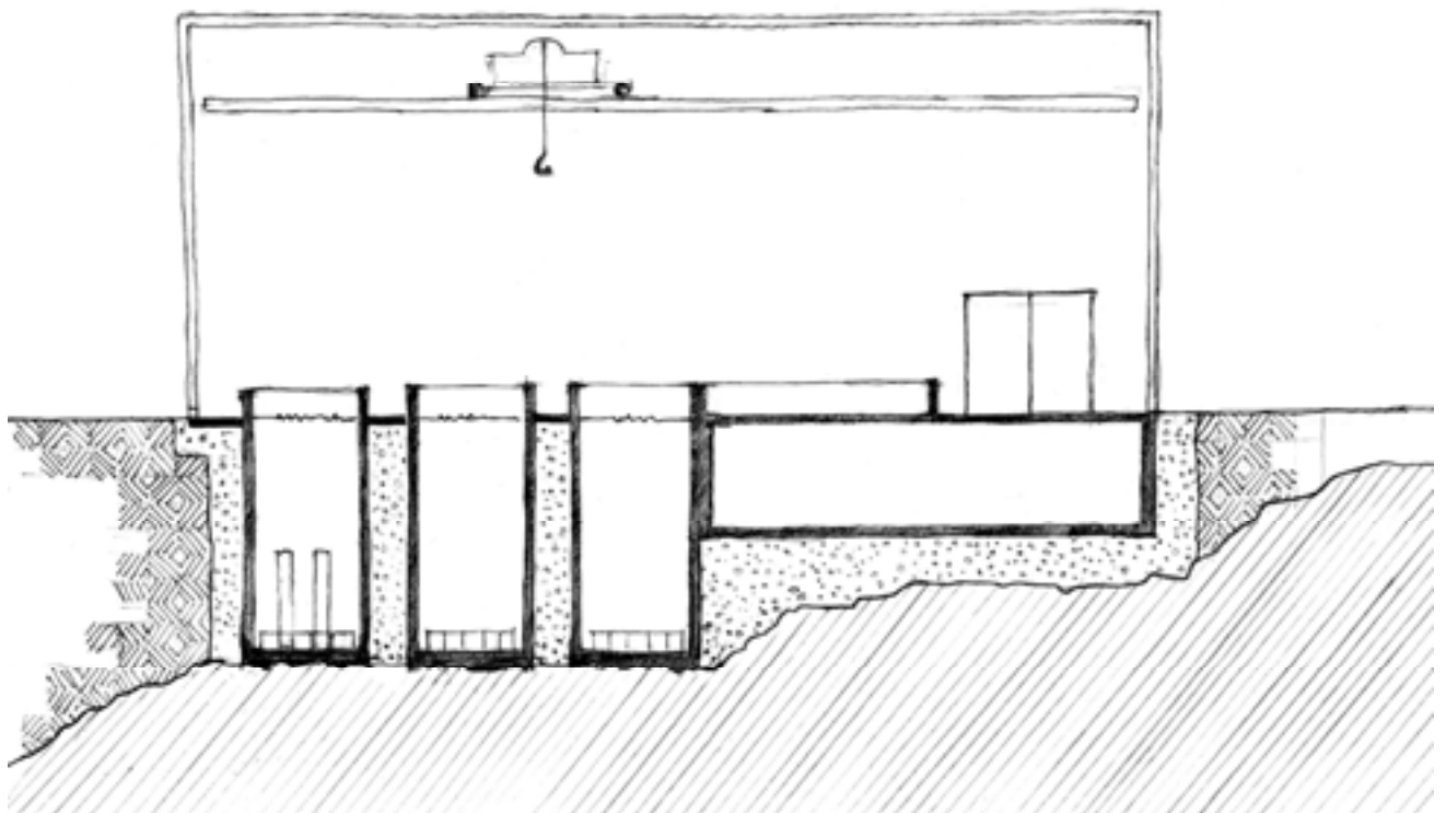
Figur 2. Sidovy av förvaringsanläggning för bränsleelement.
