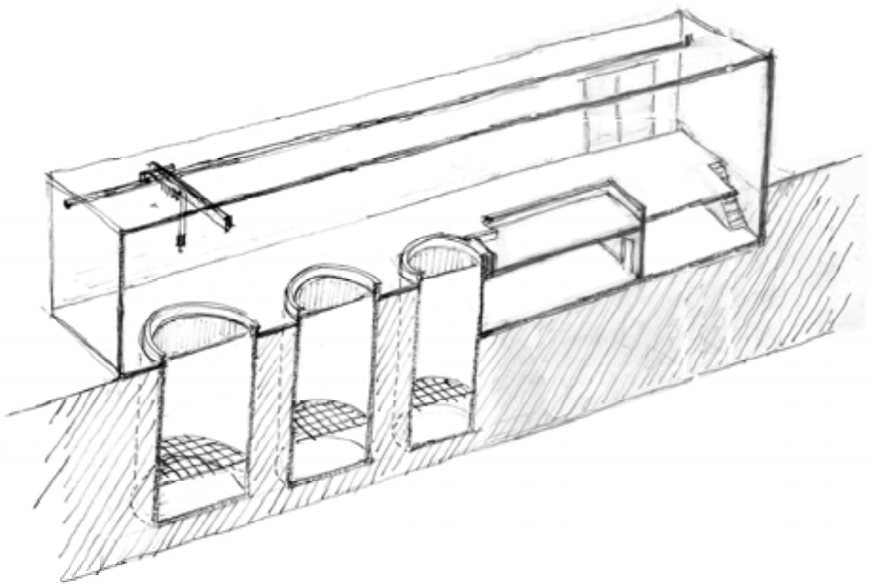
Figur 1: Översikt över Mellanförrådet för använt bränsle.
